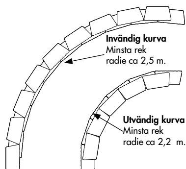
Bild 1. Invändiga och utvändiga svängda hörn/krivor.
